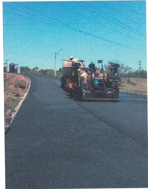
Figura 19 – Execução de camada CBUQ
