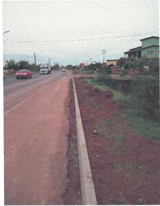
Figura 8 – Assentamento de meio fio
