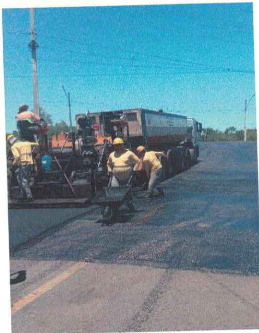
Figura 21 – Execução de camada CBUQ
