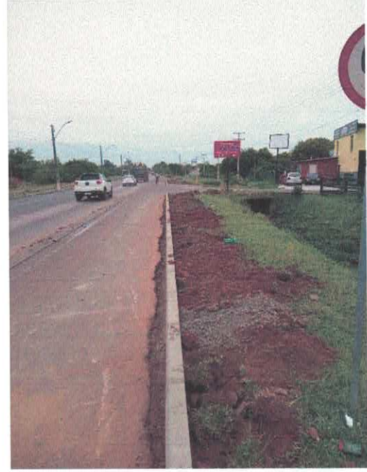
Figura 7 – Assentamento de meio fio
